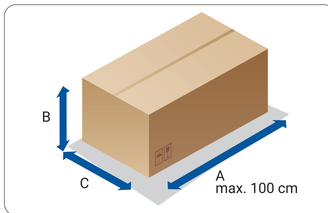
Maximální rozměry zásilky Délka: A = max. 100 cm Rozměry: A + 2B + 2C = \text{max. } 300 \text{ cm}
